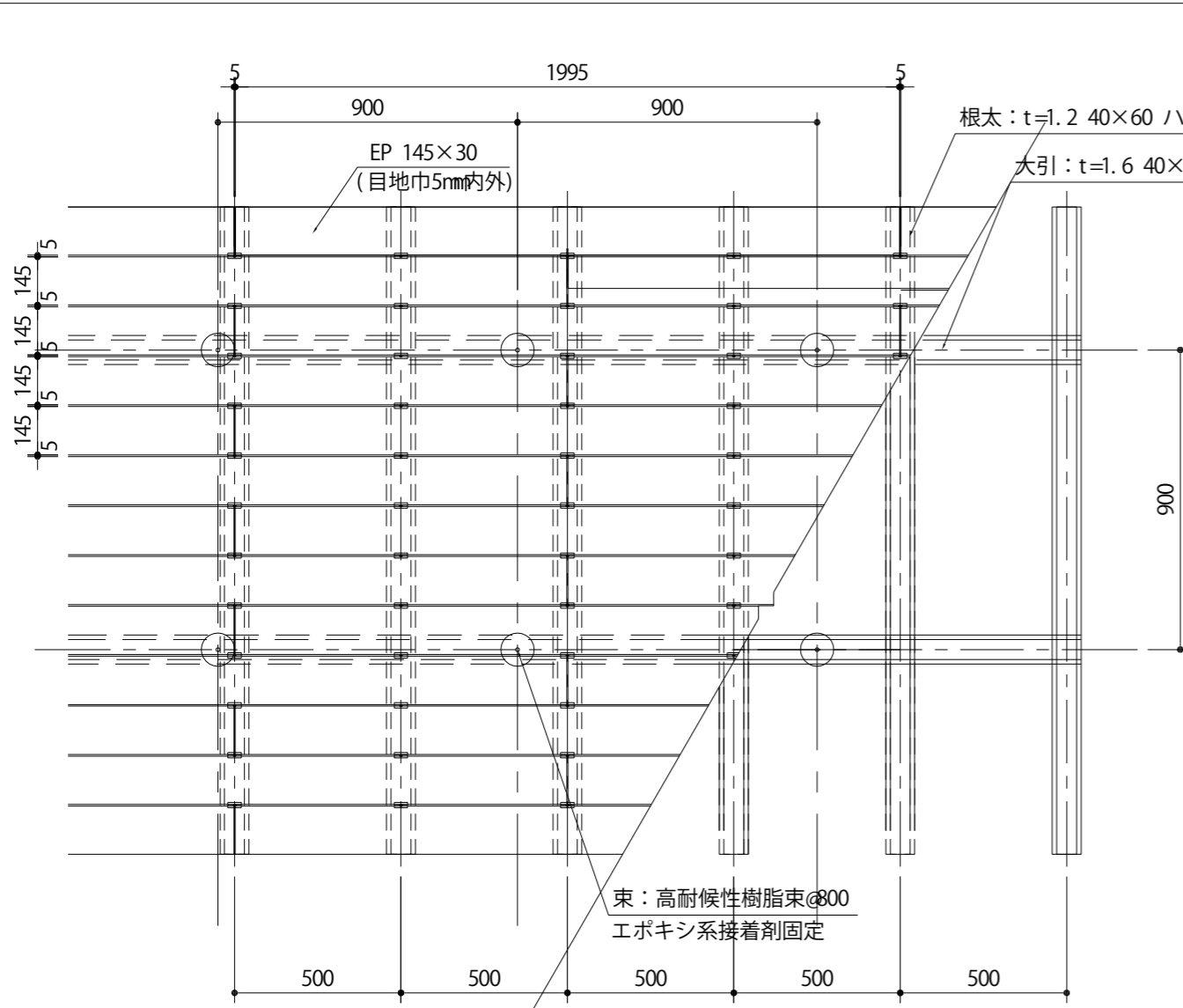
平面図 1/20
