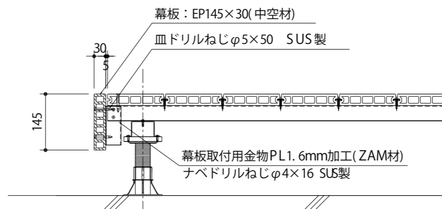
幕板取付断面図 1/10
