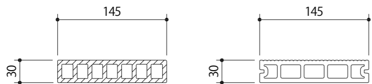
EP145×30断面形状図 1/5 (幕板用)
