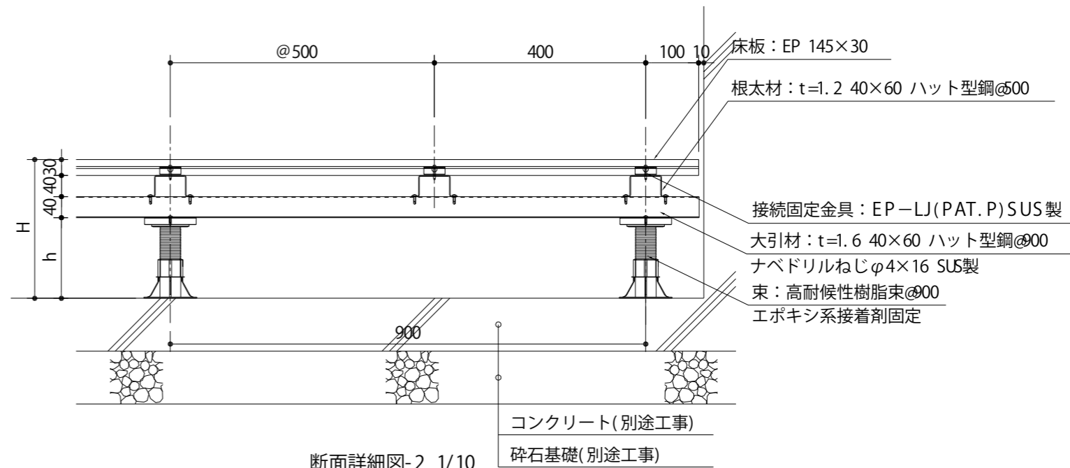
断面詳細図-2 1/10
